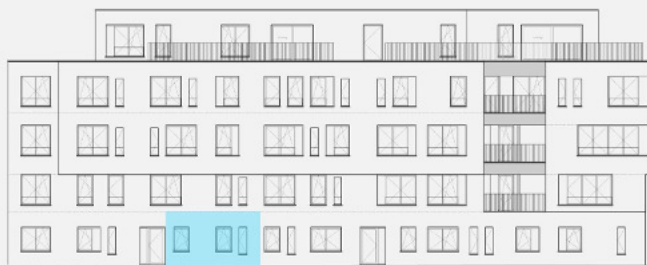
VOORGEVEL OUDE SCHAAPMARKT
