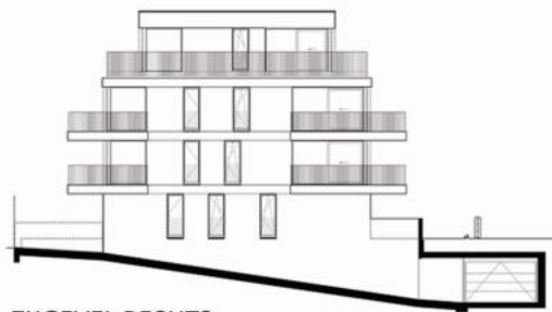
ZIJGEVEL RECHTS
