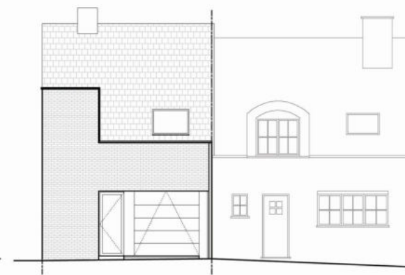
GEVEL CHICOREIERF
