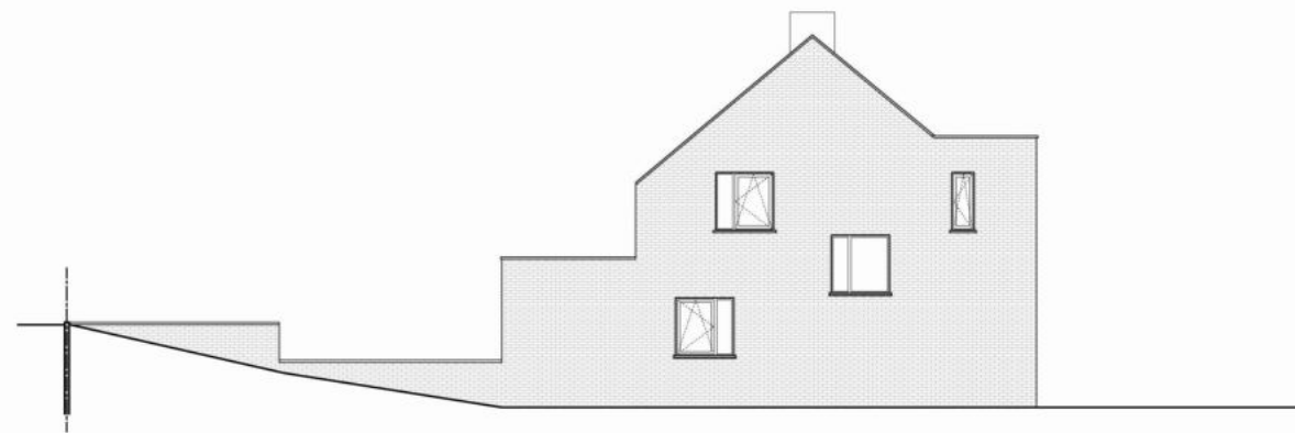
ZIJGEVEL PLEIN
